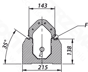
PRZEKÓJ E-E
